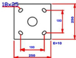
DETALLE PLACA BASE
