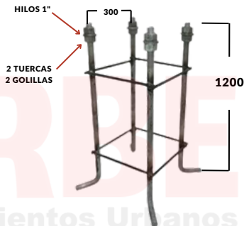
DETALLE DEL CANASTILLO
